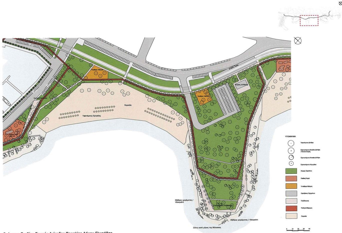
Ωρίμανση Σχεδίου Γενικής Διάταξης Παραλίας Δήμου Γλυφάδας Περιοχή Μεταξύ Μαρinas 3 και Μαρinas 4_Αποκατάσταση και Διαμόρφωση
