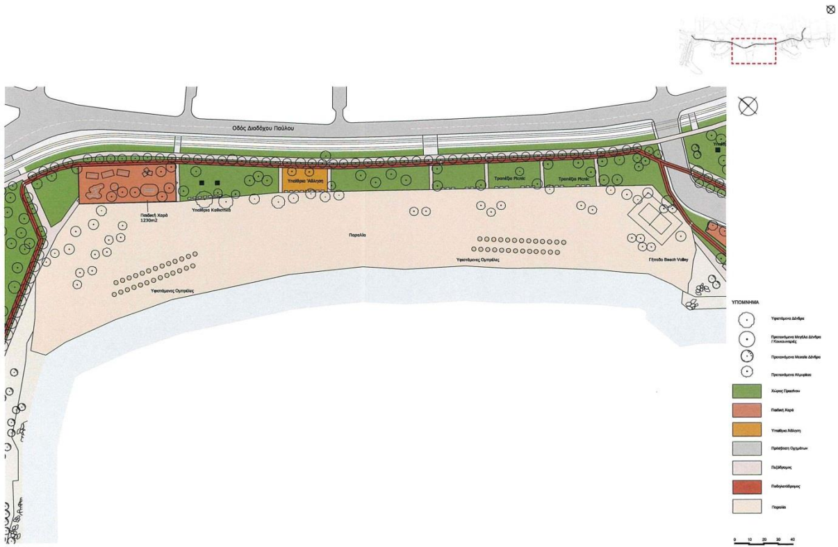
Ωρίμανση Σχεδίου Γενικής Διάταξης Παραλίας Δήμου Γλυφάδας Περιοχή Μεταξύ Μαρinas 3 και Μαρinas 4 ,Αποκατάσταση και Διαμόρφωση
