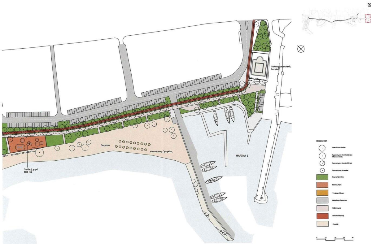
Ωρίμανση Σχεδίου Γενικής Διάταξης Παραλίας Δήμου Γλυφάδας Μαρίνα 1_Αποκατάσταση και Διαμόρφωση
