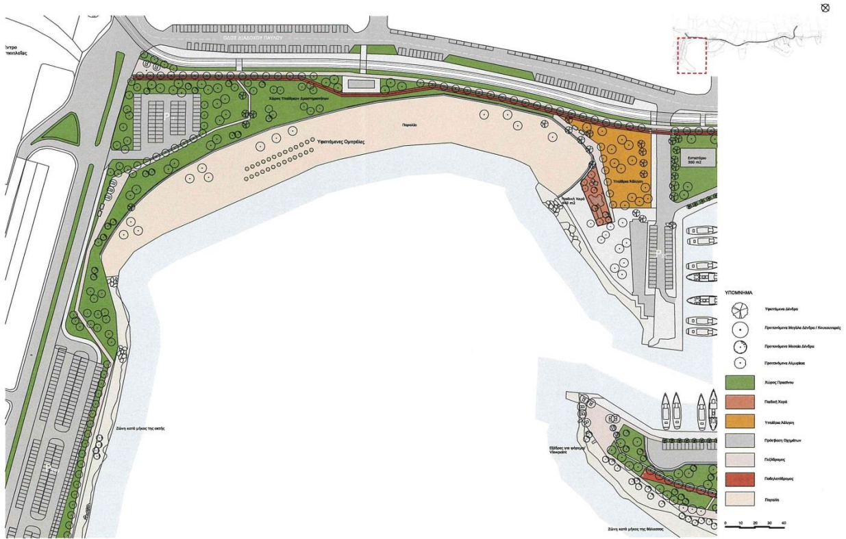
Ορίμανση Σχεδίου Γενικής Διάταξης Παραλίας Δήμου Γλυφάδας Περιοχή Βόρεια της Μαρίνας 4_Αποκατάσταση και Διαμόρφωση
