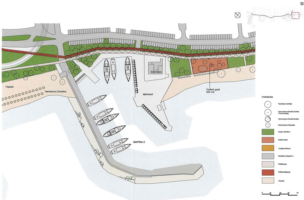
Ωρίμανση Σχεδίου Γενικής Διάταξης Παραλίας Δήμου Γλυφάδας Μαρίνα 2 και Νότια Παραλία_Αποκατάσταση και Διαμόρφωση
